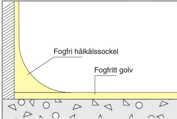
Hålkälssockel: höjd 50-200 mm, radie 30 mm.
