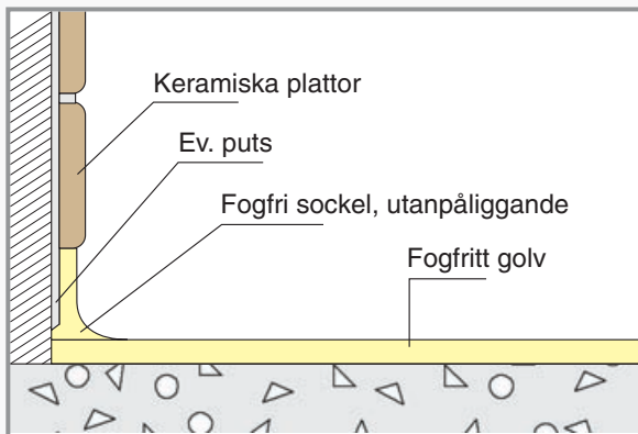
Keramiska plattor på vägg, sockelutformning. Keramiska plattor kan appliceras före sockel.
