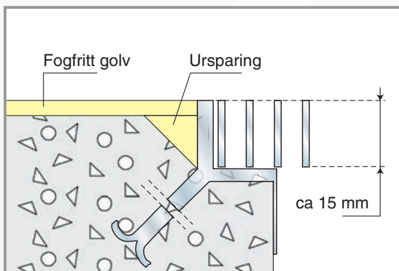
Anslutningar till brunnar, golvrännor m.m. i betong- gjutningar utförs med triangulära ursparingar mot ing- jtningsgodset. Bredd 20-50 mm, höjd 10-30 mm.
