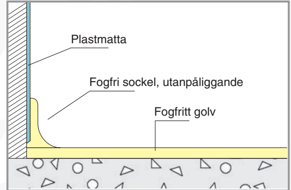
Plastmatta på vägg, sockelutformning.
