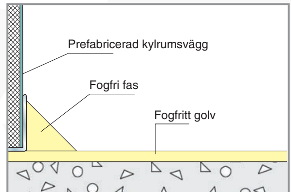
Anslutning mot prefabricerad kylrumsvägg. Fas: bredd 20-30 mm, höjd 20-30 mm.
